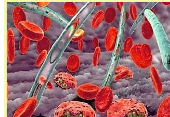
طفيلي وحيد الخلية بلازموديوم يسبب مرض الملاريا بتدمير الكريات الدموية الحمراء
